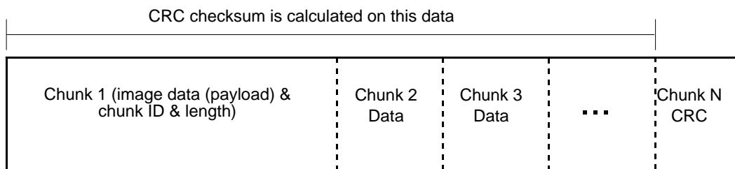
Fig. 115: CRC Checksum
