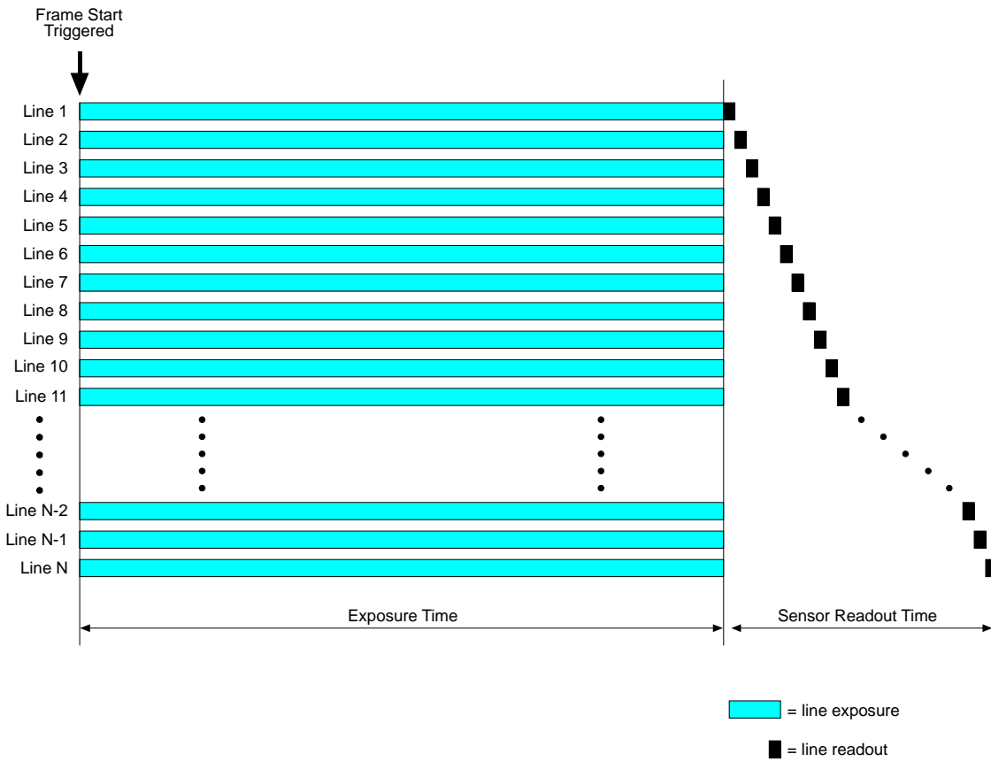
Fig. 60: Global Shutter
